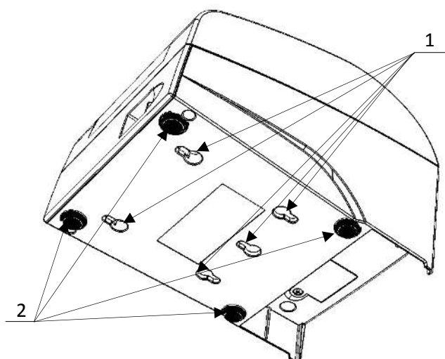
Рисунок 5. Крепление ПД
